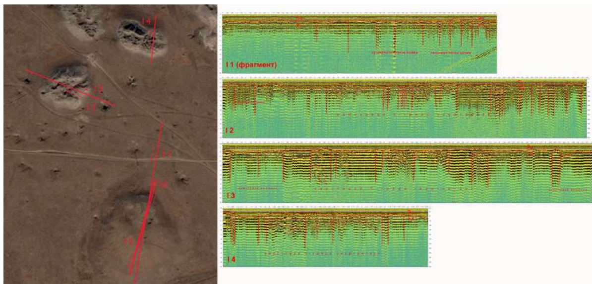
Рисунок 4 – Размещение трасс профилей на участке «Карстовые гряды» (Индерский соляной купол) и интерпретация георадарных профилей
